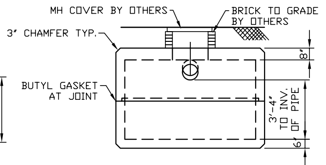
ELEVATION A-A
